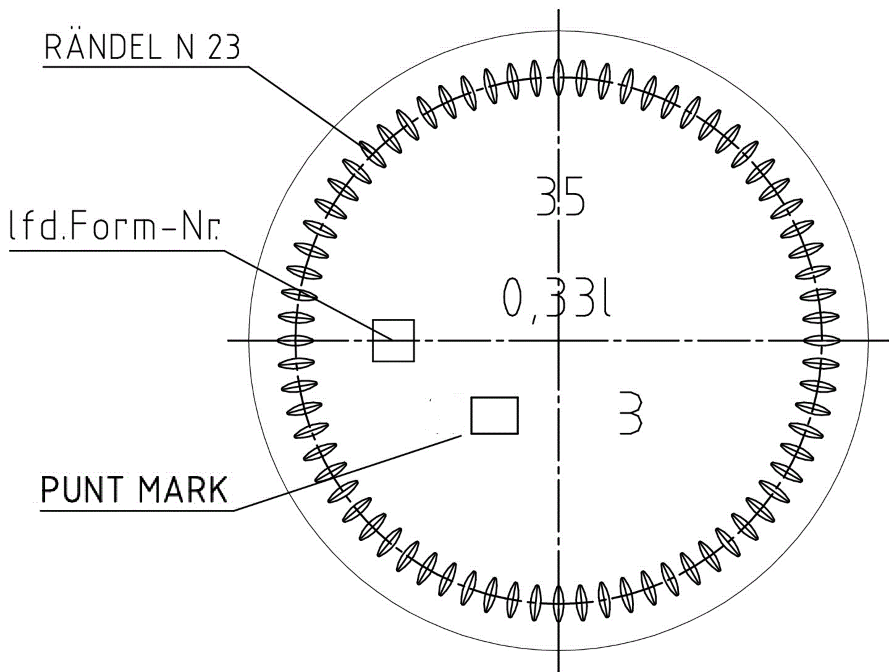
Bodenansicht
