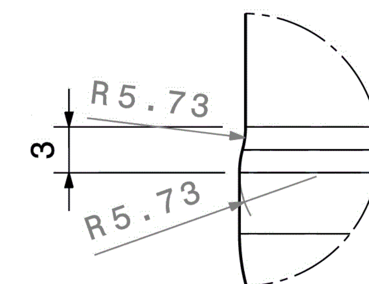
Detail C Maßstab: 2:1
