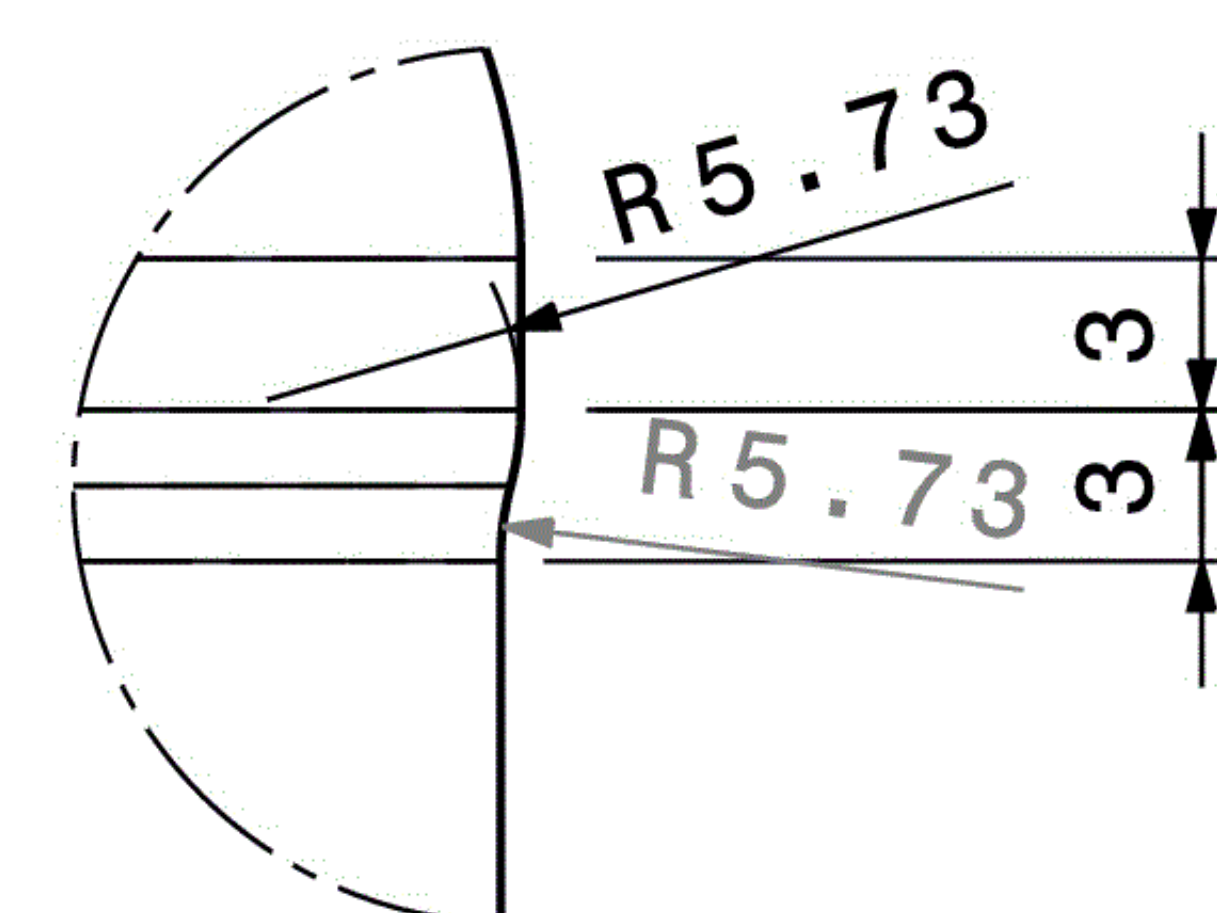
Detail A Maßstab: 2:1
